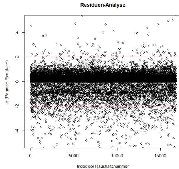
Abbildung 6.2: Standardisierte Residuen (e.D.)
